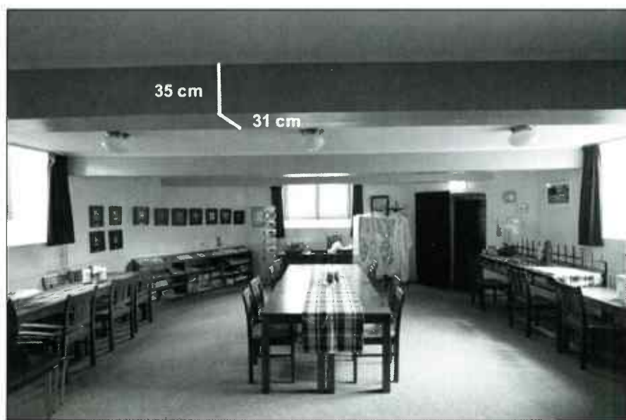
Consistorie. De 4 balken die het balkon dragen, zijn tenminste 35 bij 31 cm dik
