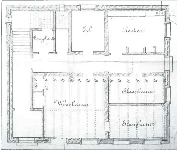
Bouwtekeningen van het kantongerecht te Zuidhorn uit 1882 Boven: begane grond met dienstwoning en cel. Onder : verdieping met gerechtszaal en kamers voor rechter en griffier.
