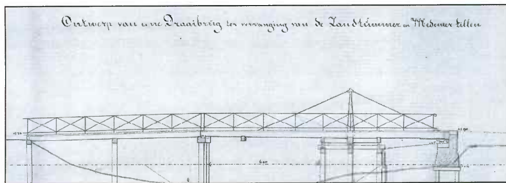
Fig. 5 In 1858 werden twee tillen over het Hoendiep tussen Gaarkeuken en Noordhorner-tolhek vervangen door een draaibrug. In de cirkels: links de Medenerhellingtil, rechts de Zandumer til. Daartussen, en oostelijk van het Kleine Diep, de nieuwe draaibrug die later Saartjesdraai werd genoemd, naar brugwachter en scheepsjager Jan Saartjes.
